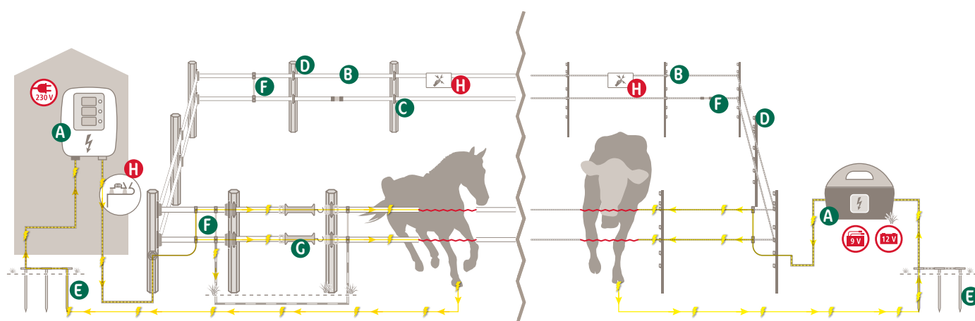
Gard permanent cu tensiune de alimentare 230 volţi
